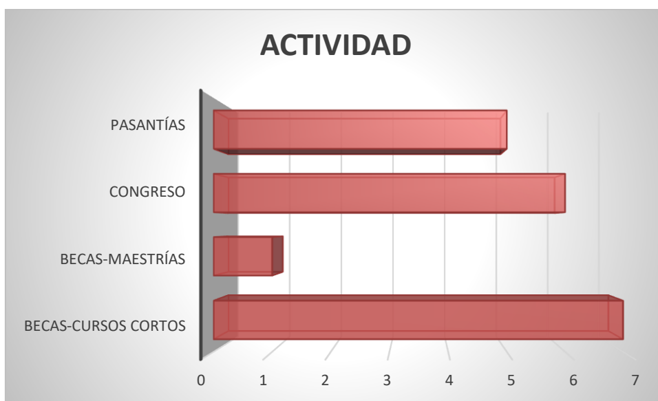
Gráfico 1. Actividades realizadas
