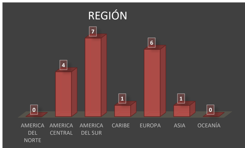
Gráfico 2. Región
