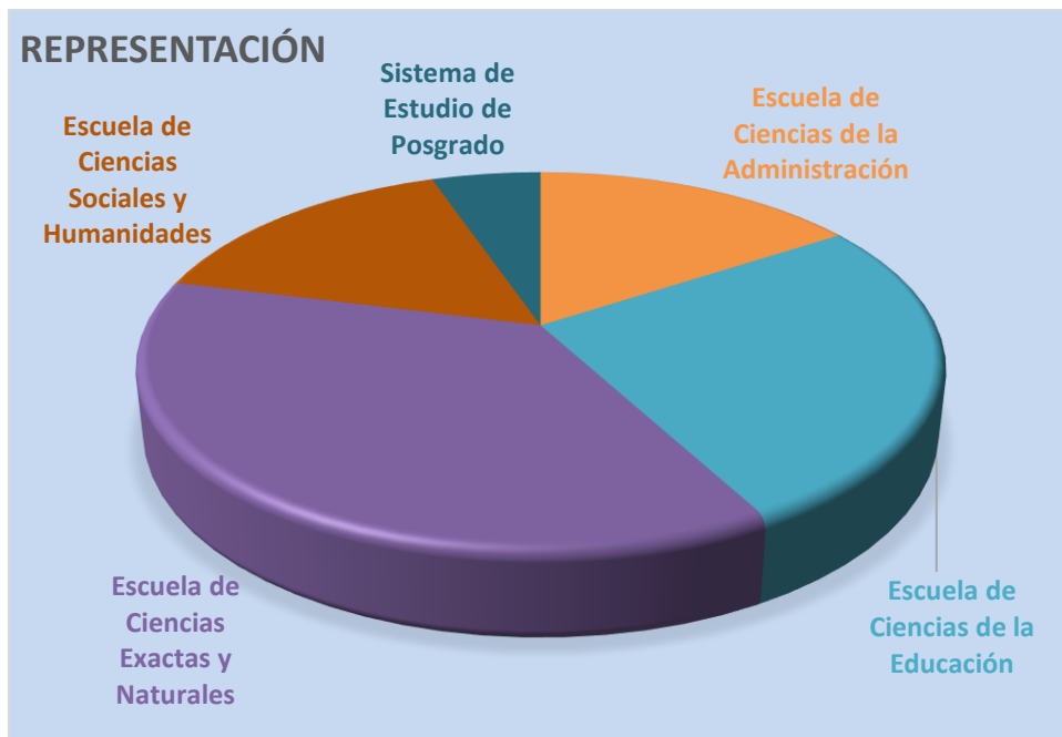
Gráfico 3. País
